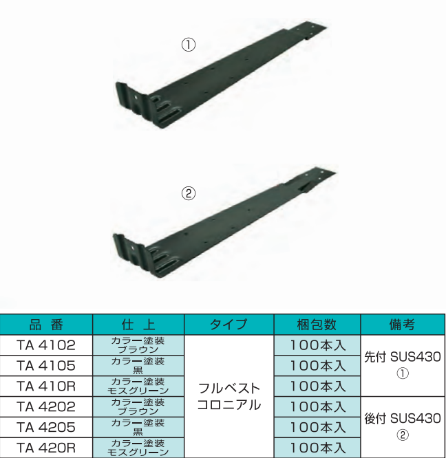
扇型 雪止め金具
