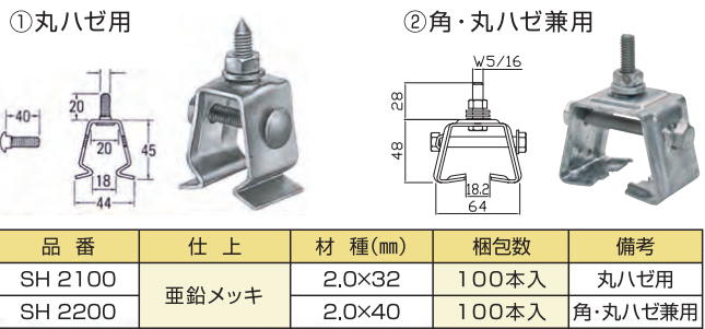
屋根上金具
