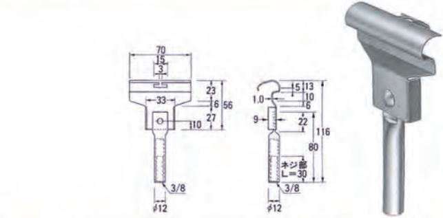
丸ハゼ吊子
