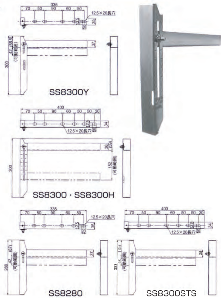
鼻かくし取付金具 ZAM ® ・スーパーダイマ ® ステン
