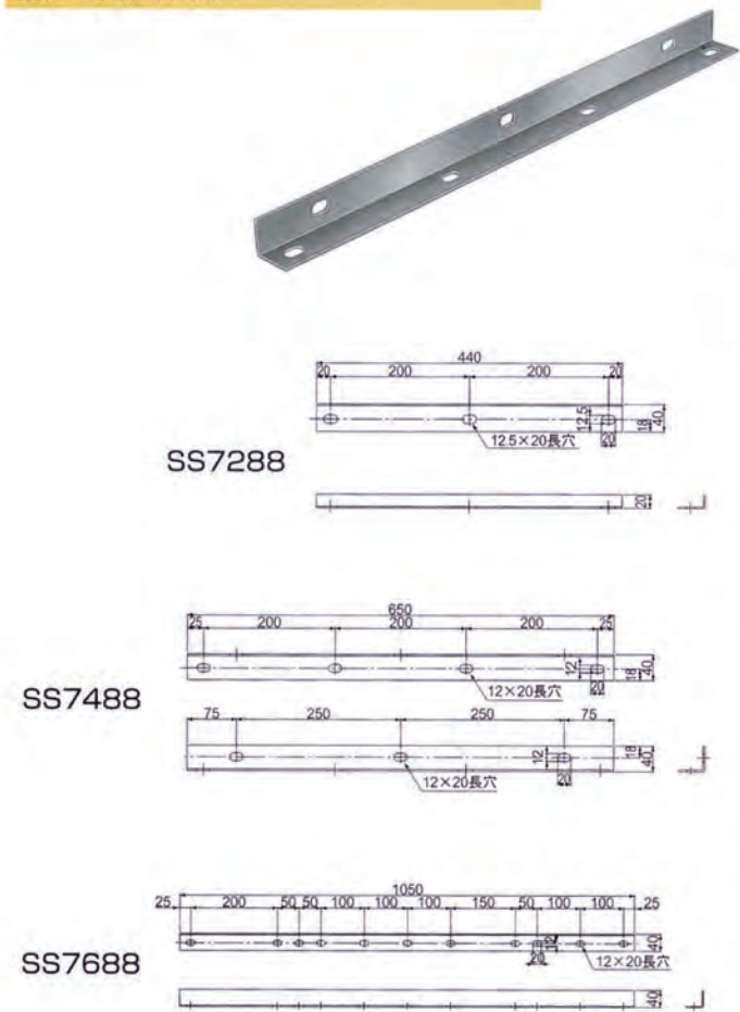
妻アングル ZAM ®
