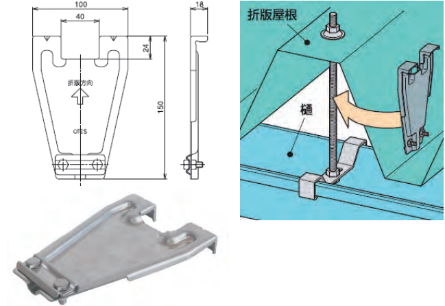
吊ボルト補強プレート PAT.P ステン・ZAM ®
