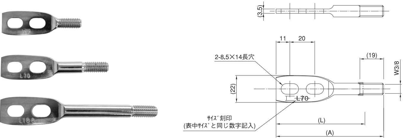
ステン モダンボルト二つ穴
